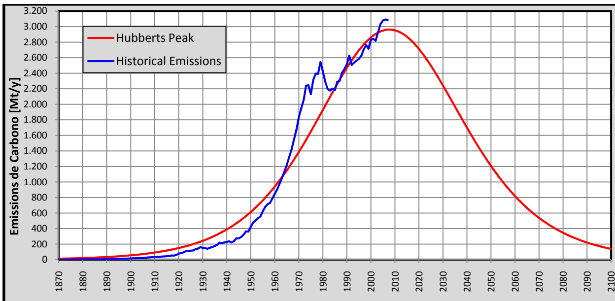
Gráfico 8: Curva de Hubbert de las emisiones mundiales de carbono por los combustibles líquidos fósiles
